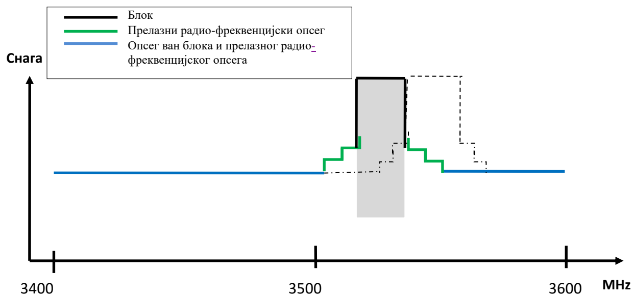
Слика 2. Илустрација ВЕМ ( Block Edge Mask ) у случају синхронизованих мрежа
