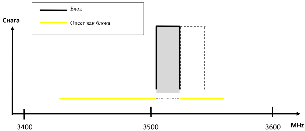
Слика 3. Илустрација ВЕМ ( Block Edge Mask ) у случају несинхронизованих и полусинхронизованих мрежа
